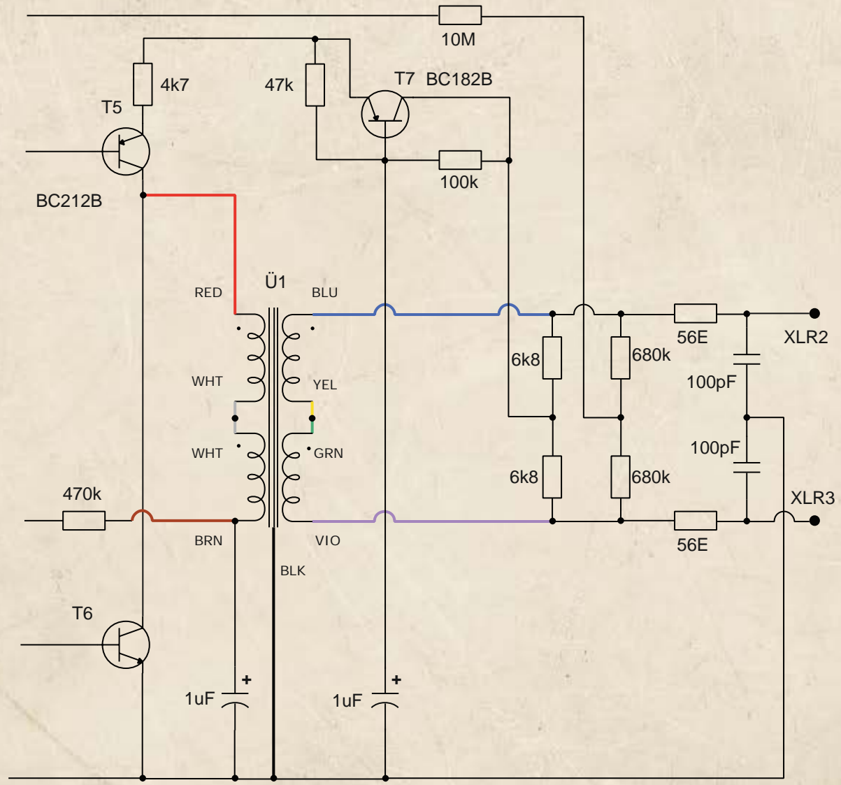
Ü1 / 90 331 transformer
